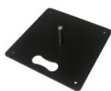
Płaska stal malowana proszkowo waga: 4kg wymiar: 400 x 400 mm
